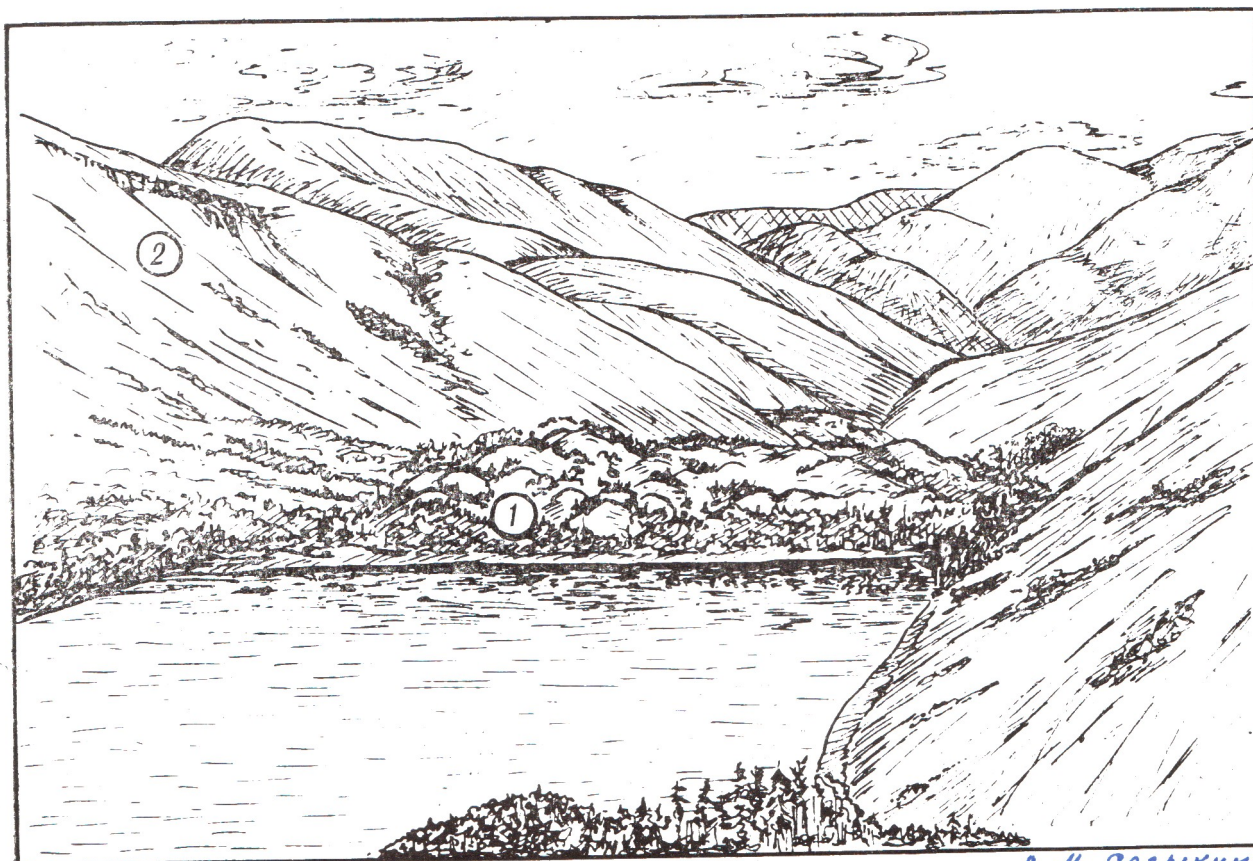
Рис. 1. Вид с юго-запада на сейсмогравитационный обвал Омот (рисунок с фото А. М. Созыкина Ю. К. Иващенко). 1 — аккумулятивное тело обвала; 2 — стенка отрыва.
