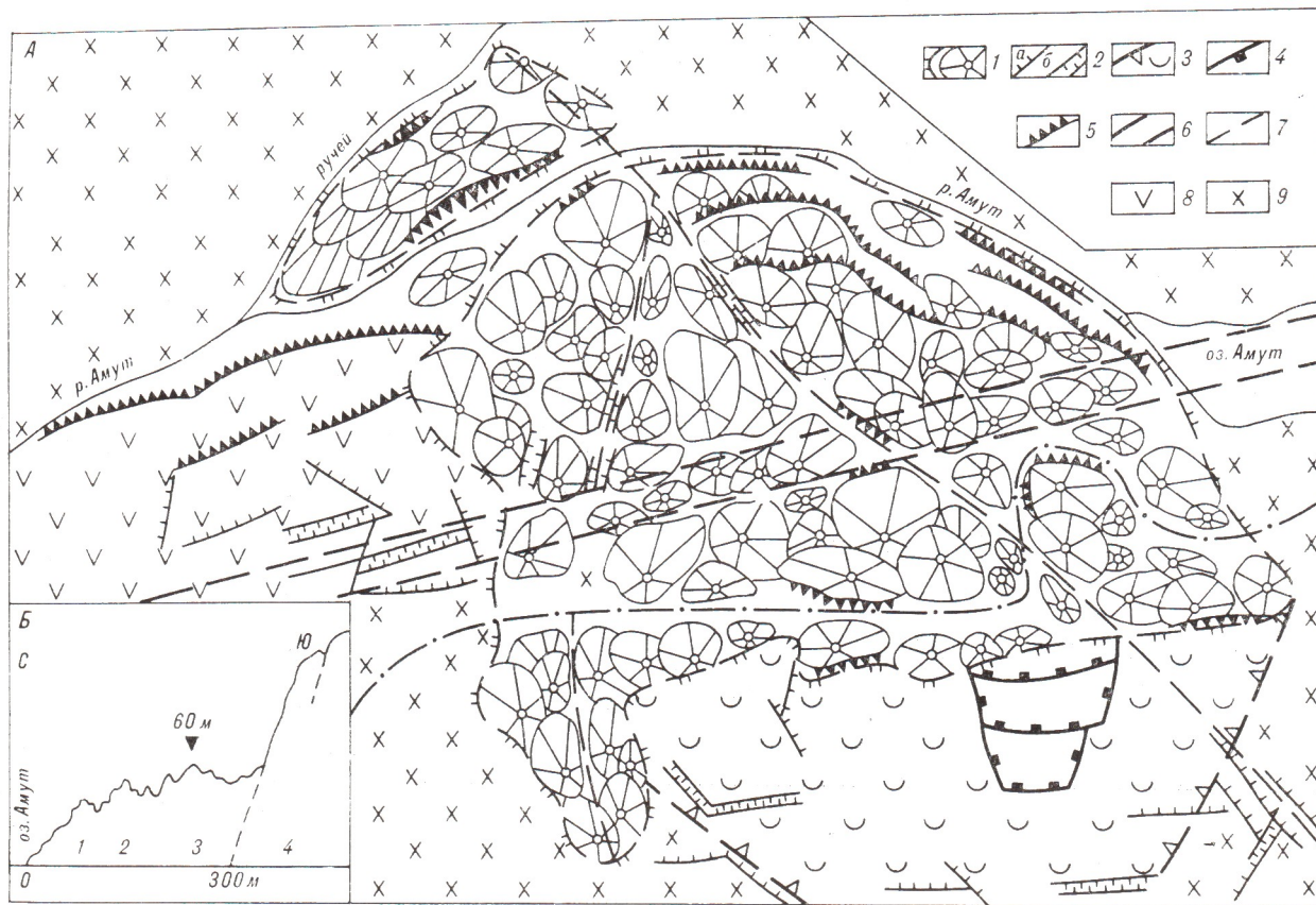
Рис. 4. Плановая схема Амурской сейсмогравитационной структуры. А: 1 — граница аккумулятивного тела обвала и отдельные купола на нем; 2 — тектонические уступы (а) и рвы (б); 3 — стенка отрыва; 4 — экзогенные уступы, ограничивающие оползни; 5 — эрозивно-тектонические уступы; 6 — Амурская зона разломов; 7 — поперечные разломы; 8 — блок пород, вовлеченный в опускание, но сохранивший первоначальную структуру; 9 — склоны Амурской долины. Штрихпунктиром показано положение грунтовой дороги в пределах обвала. Б — обобщенный профиль через Амурский обвал: 1, 2 — вала аккумулятивного тела первой генерации; 3 — вал второй генерации; 4 — стенка отрыва (составил Ф. С. Онухов).
