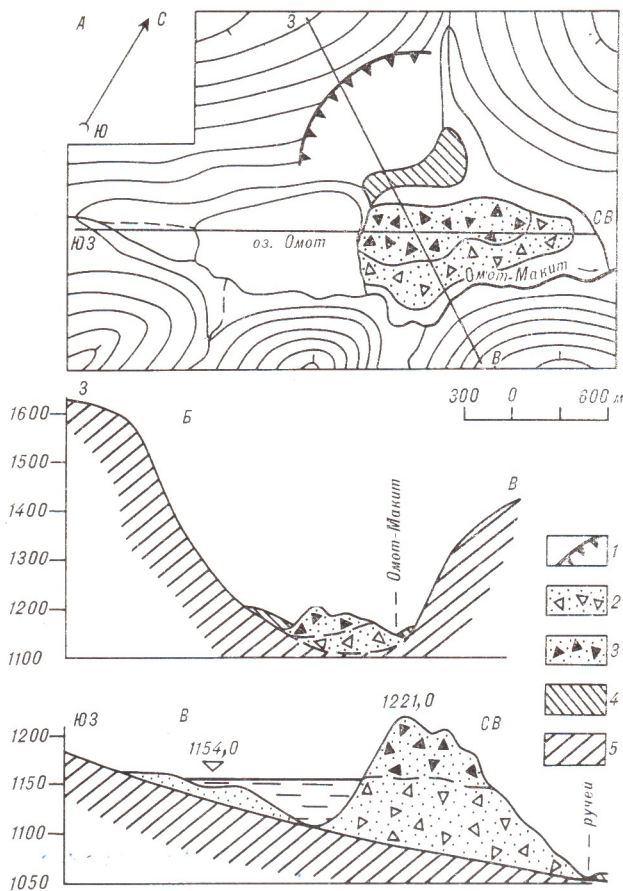
Рис. 2. Плановая схема сейсмогравитационной структуры Омот (А) и разрезы по профилям (Б, В') (составили Ю. К. Ивашинников и А. М. Сазыкин). 1 — стенка отрыва обвала; 2 — смещенный материал генерации первого землетрясения; 3 — то же, генерации повторного землетрясения; 4 — щебнисто-глыбовый материал в стадии смещения; 5 — коренные породы верхнемелового возраста: туфы липаритов и дацитов.
